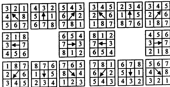
(a) 좌수법 (b) 우수법 그림 6: 경계 추적을 위한 우선순위
