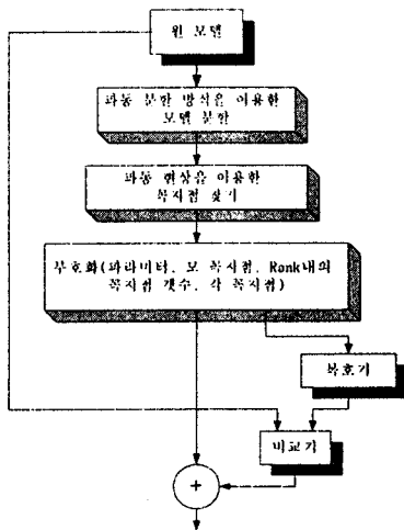
그림 7. 부호화 흐름도
