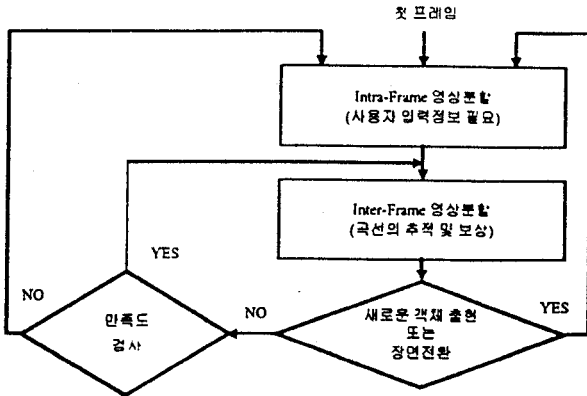
그림 1. 반자동 영상분할 알고리즘
