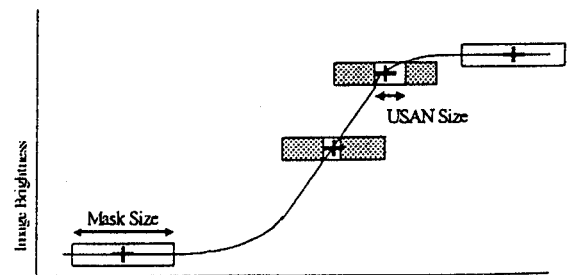
그림 2. SUSAN 알고리즘
