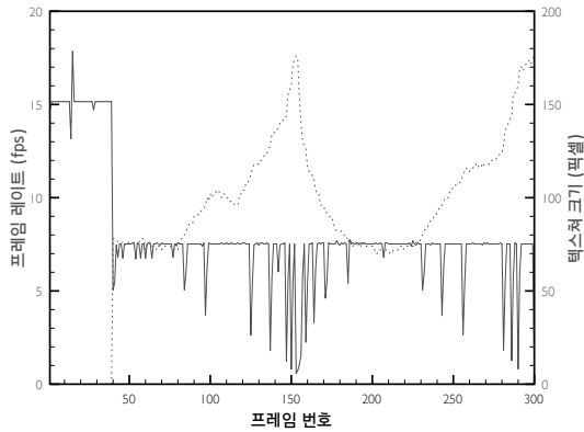
그림 12: 텍스처 크기에 따른 프레임 레이트 변화
