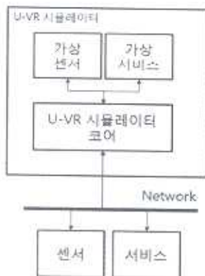
그림 4. U-VR 시뮬레이터 구조
