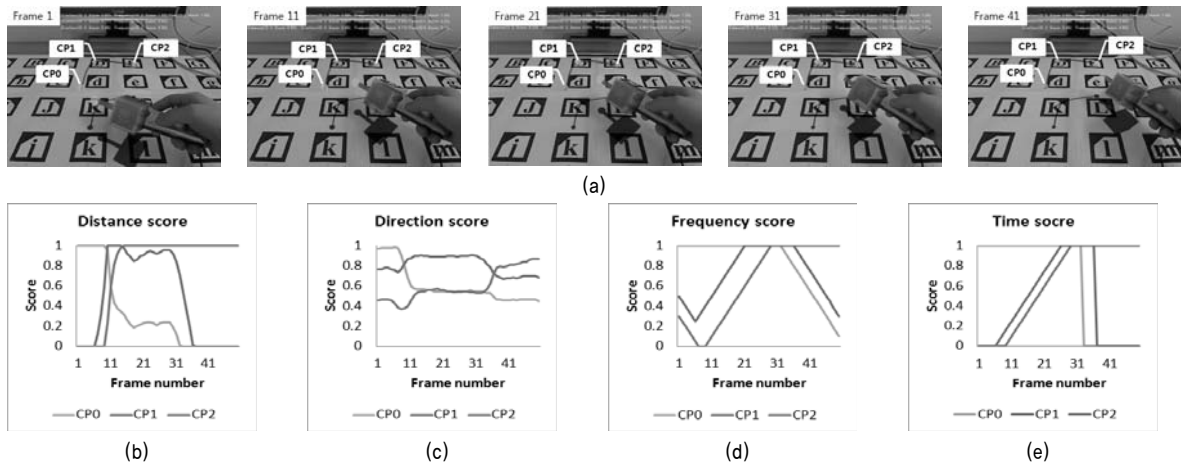
그림 9. 이동 궤적의 조정점 선택을 위한 스코어 측정의 예시: (a) 총 50 프레임 동안의 테스트 이미지 시퀀스 (10 프레임 간격으로 정지 영상을 표시함); (b) 거리 스코어; (c) 방향 스코어; (d) 빈도 스코어; (e) 시간 스코어.
