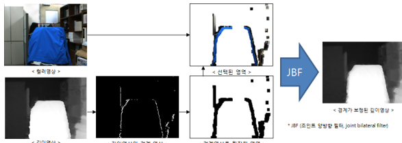
그림 9. 컬러영상과 깊이영상간의 경계 보정 Fig. 9. Object boundary compensation
